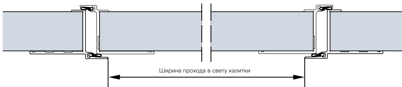
Конструкция калитки секционных ворот со строительной глубиной 42 мм
